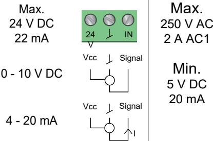
Wiring, analog input
