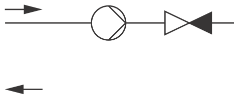
Fig. 4 Válvula antirretorno
