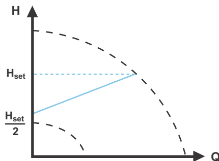
Fig. 28 Pression proportionnelle
