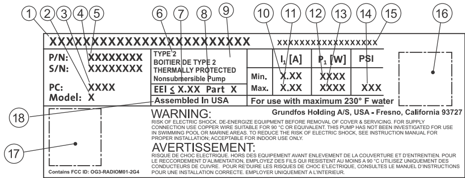
Fig. 5 Ejemplo de placa de características
