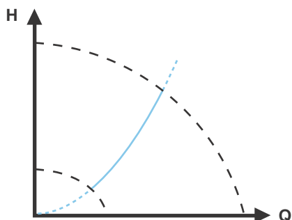
Fig. 30 Temperatura constante
