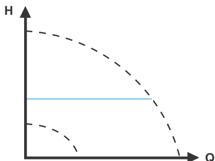
Fig. 29 Presión constante
