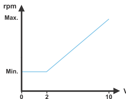
Fig. 37 Función punto de ajuste externo, 0-10 V
