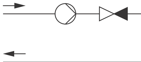
Fig. 4 Clapet anti-retour
