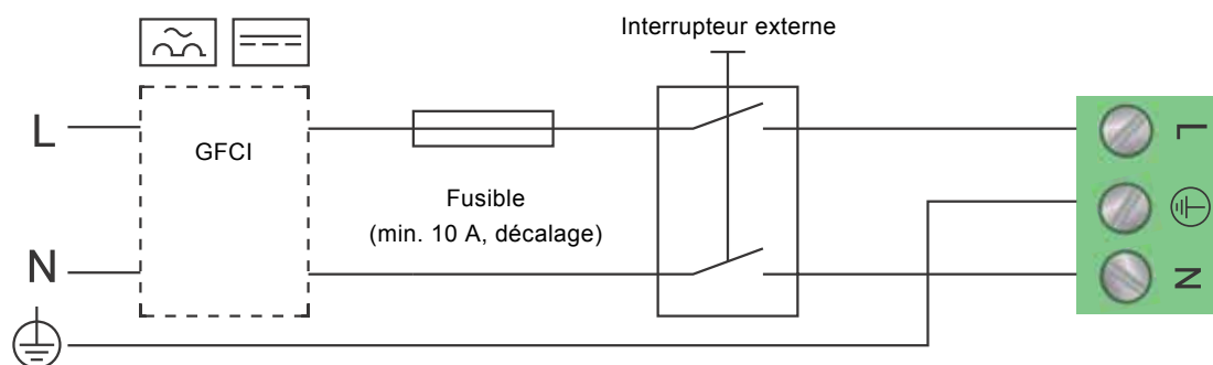
Fig. 14 Exemple de connexion traditionnelle, 1 x 230 V \pm 10 %, 50/60 Hz
