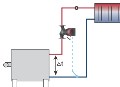
Fig. 32 Température différentielle
