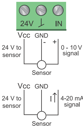
Fig. 20 Câblage, entrée analogique
