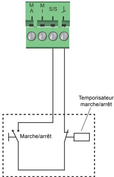
Fig. 18 Entrée digitale
