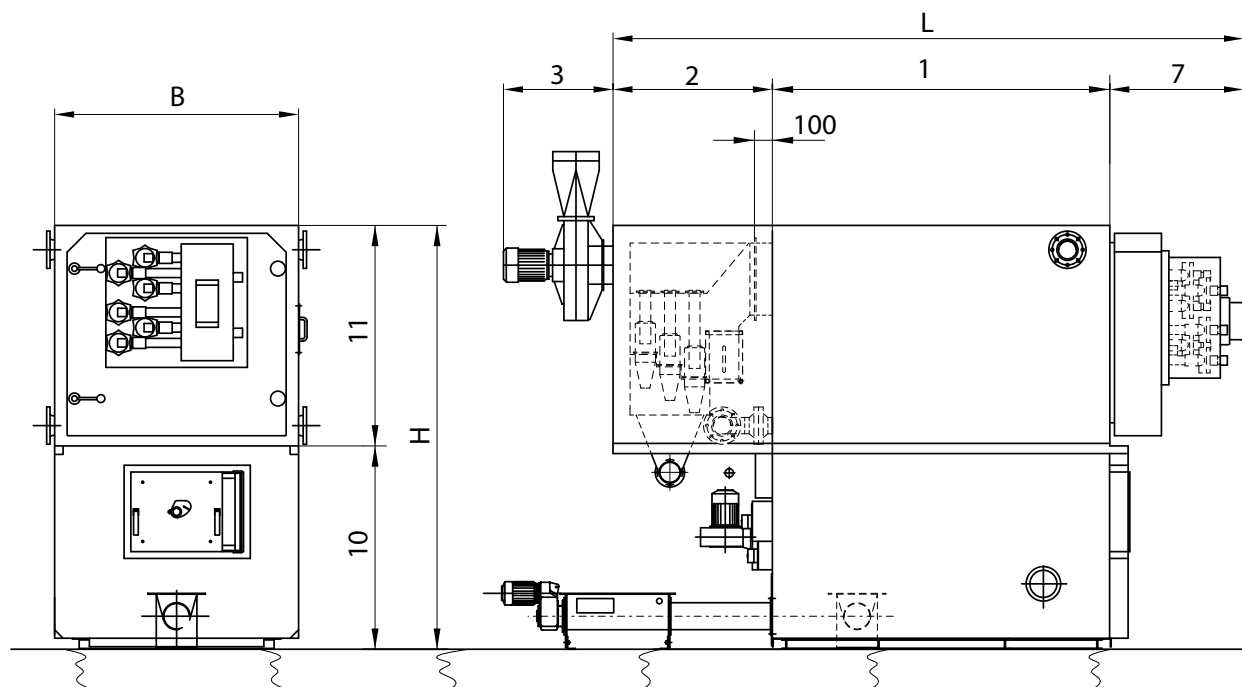
Fig. 12 Dimensions
