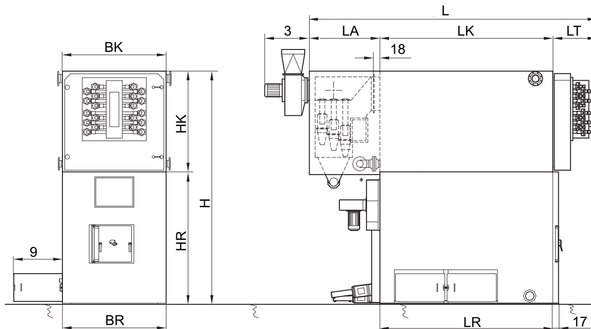
Fig. 14 Dimensions
