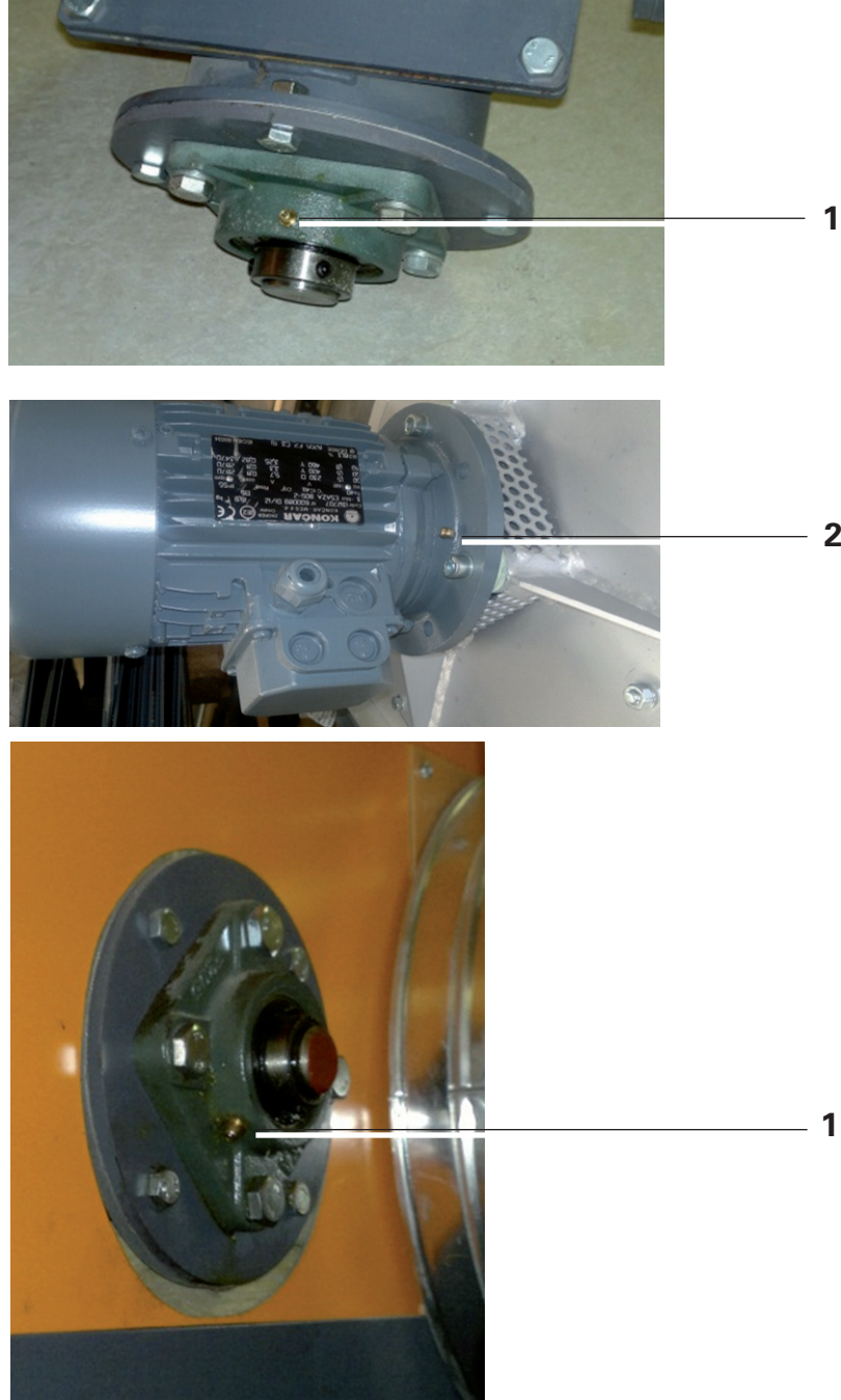
Fig. 21 Lubrication points
